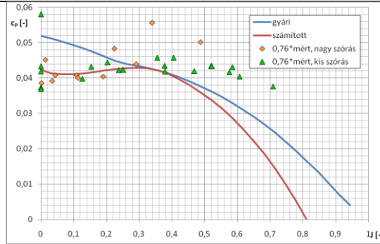
5. ábra A mért és számított légszár karakterisztika [1]
