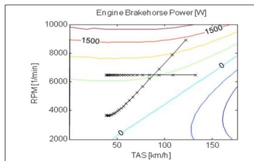
6. ábra A légszár munkaponti fordulatszáma a repülési sebesség függvényében
