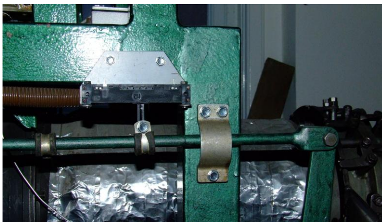
14. ábra. A fűvócső keresztmetszetét rögzítő toló potenciométer
