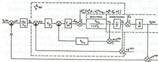
1. ábra Az irányszög robotpilóta hatásvázlata
