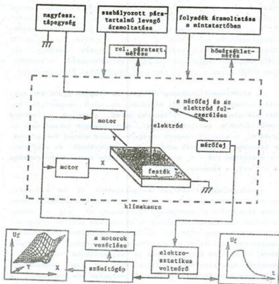
1. ábra A kísérlet összehallítása
