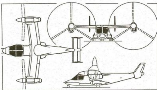
1. ábra Bell XV-15 háromnézetű rajza
